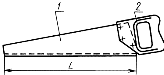
1 — полотно, 2 — ручка
